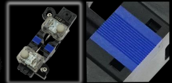
对应间隔 250µm 的光纤
